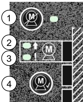
Abbildung 7 - Motorbedienfeld
