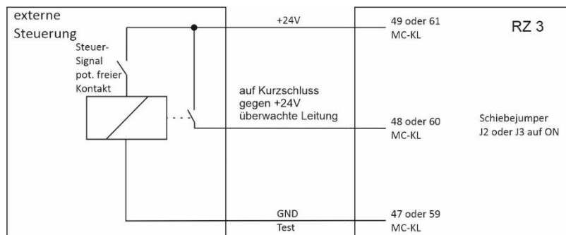
Beispiel 1: mit potentialfreiem Kontakt einer externen Steuerung
