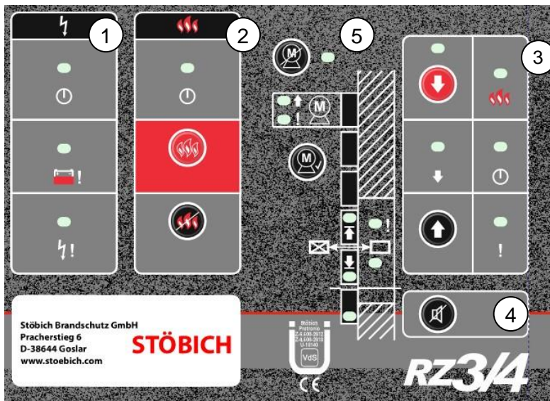
Abbildung 1 - Anzeige- und Bedienelemente der Feststellanlage (Steuerung) Typ RZ3
