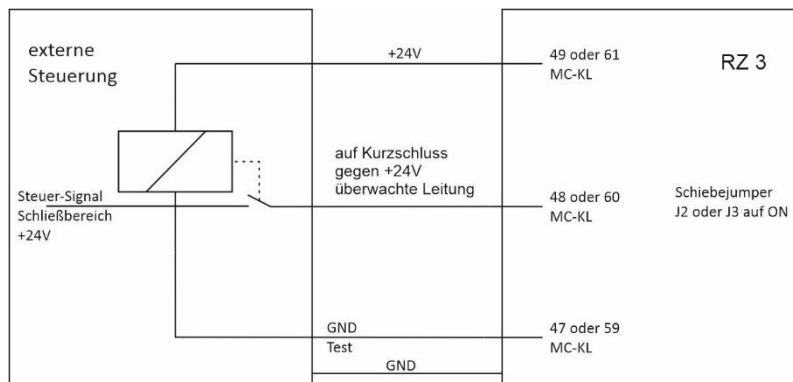
Beispiel 2: mit potentialbehafteten 24V Signal einer externen Steuerung
